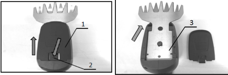
1. Μυστικά? 2. Κουμπί του μυστικού · 3. Λεπίδες διάτμησης.
